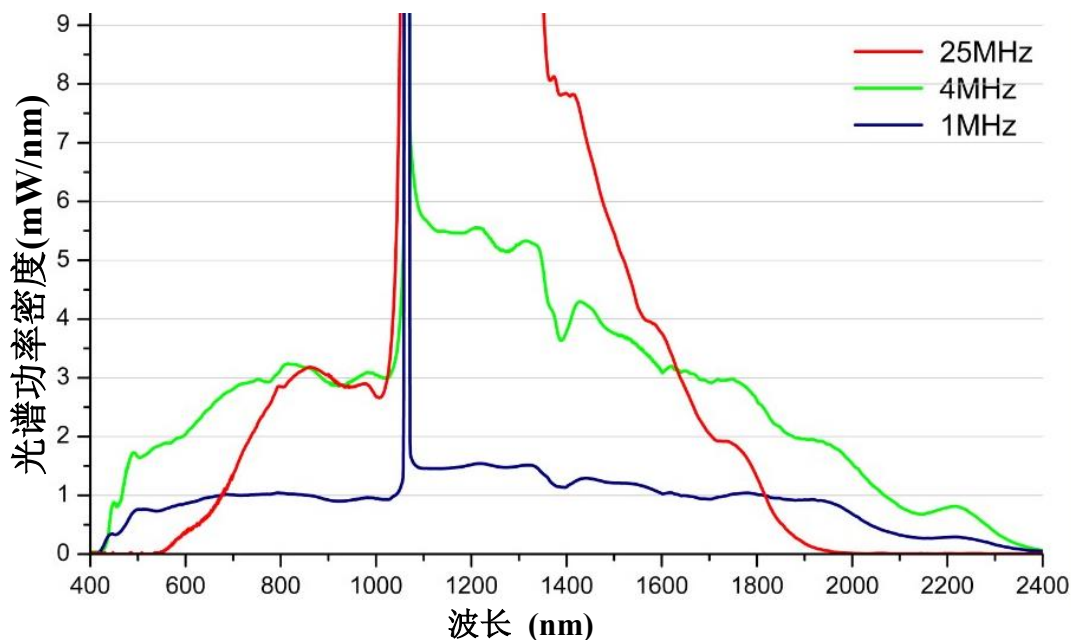
6W SC-PRO-的典型光谱
